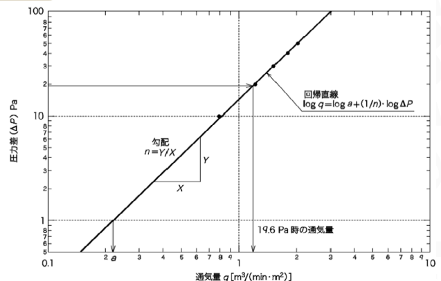
壓力差與洩漏量線性關係圖
