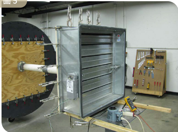
排煙閘門氣密性檢測實景（由陽鼎實業股份有限公司專業提供）
