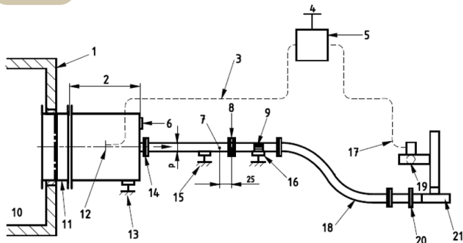
EN1366-10 氣密洩漏量檢測裝置示意圖
