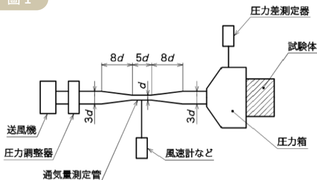
日系氣密性檢驗裝置示意圖
