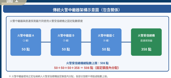
傳統火警中繼器架構示意圖（包含關係）
