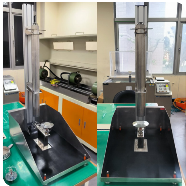
護罩橫向衝擊試驗
