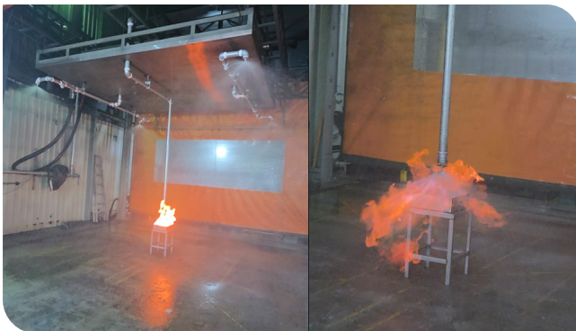
橫向撒水試驗 (感熱元件未動作前)
